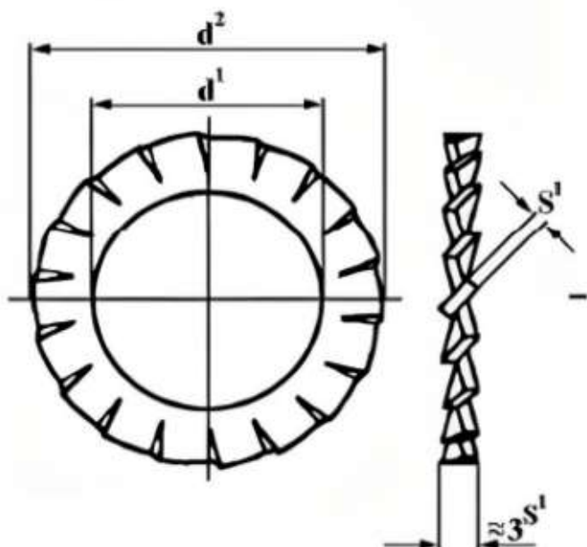
FORMA A DENTADO EXTERNO
